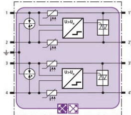
Prinzipialschaltbild BXTU ML4 BD 0-180
