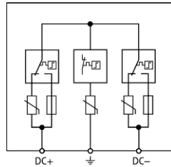
Prinzipialschaltbild DCU YPV SCI 1000 1M
