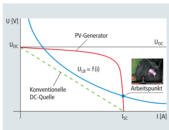
Bild 5 Quellenkennlinie einer konventionellen DC-Quelle vs. der eines PV-Generators; beim Schalten von PV-Quellen wird der Bereich der Lichtbogenbrennungsspannung durchlaufen
